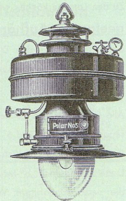
POLAR-Lampe Nr. 5 a 800 - 1000 HK. Behälterinhalt 3 Ltr. Petroleumverbrauch \frac{1}{6} Ltr. Höhe 51 cm Gewicht 5,5 kg Durchmesser 32 cm
